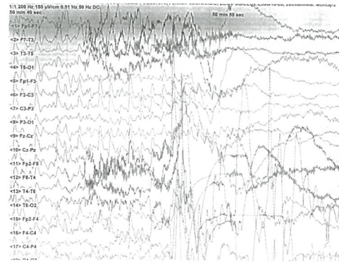
Şekil 2b. Takiben jeneralize diken dalgı deşarjları
