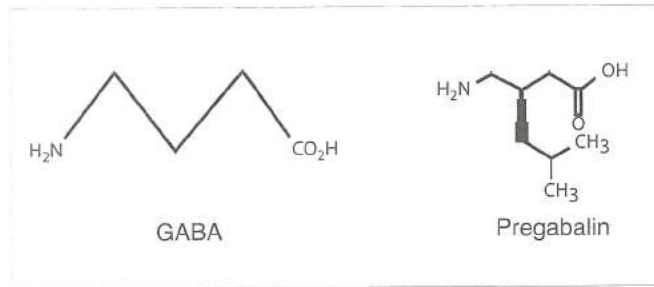
Şekil 1. GABA ve pregabalinin kimyasal yapıları [Martin 1999 (Kaynak 4) & Kavoussi 2006'dan (Kaynak 1) adapte edildi]
