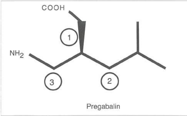
Şekil 2. Yapı-aktivite ilişkisi çalışmalarında pregabalin kimyasal yapısının pek çok yan-zincir elemanlarının stereokimyasal oryantasyonu bileşiğin farmakolojik aktivitesi ile sonuçlanır [Guay 2005'ten (Kaynak 6) adapte edildi]
